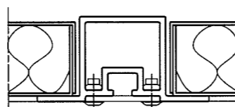
A - A PROFIL NITAS I FLÄNS MED STÅLNIT Ø4.0 BN01-0512
