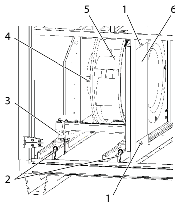
Exempel fläktenhet storlek 10-16
